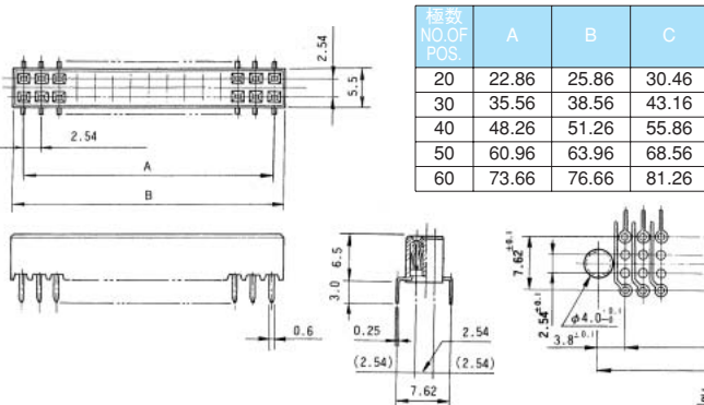
基板穴配列図
