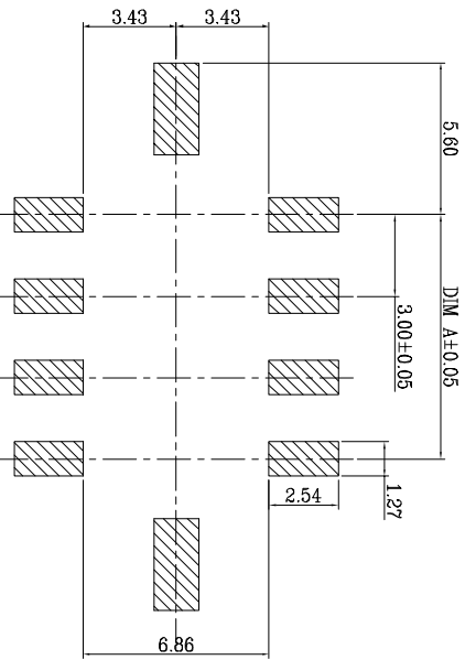
P.C.B Layout
