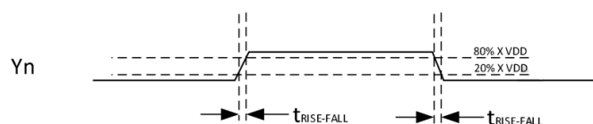
图10 上升和下降时间 t_{RISE-FALL}
