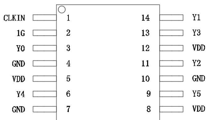
图3 HAC1106TS 引出端排列图（顶视图）
