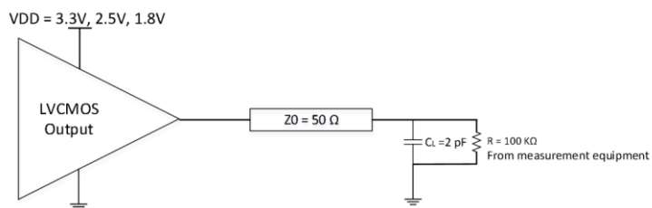
图4 测试负载电路
