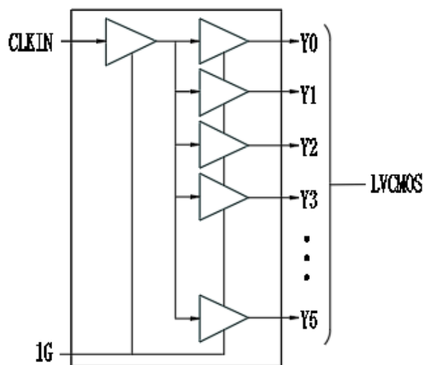
图1 功能框图
