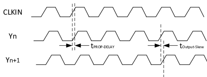
图9 传播延迟 t_{PROP-DELAY} 和输出偏斜 t_{Output-SKEW}
