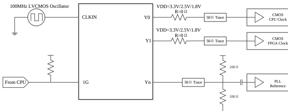
图11 HAC1106TS 典型应用图
