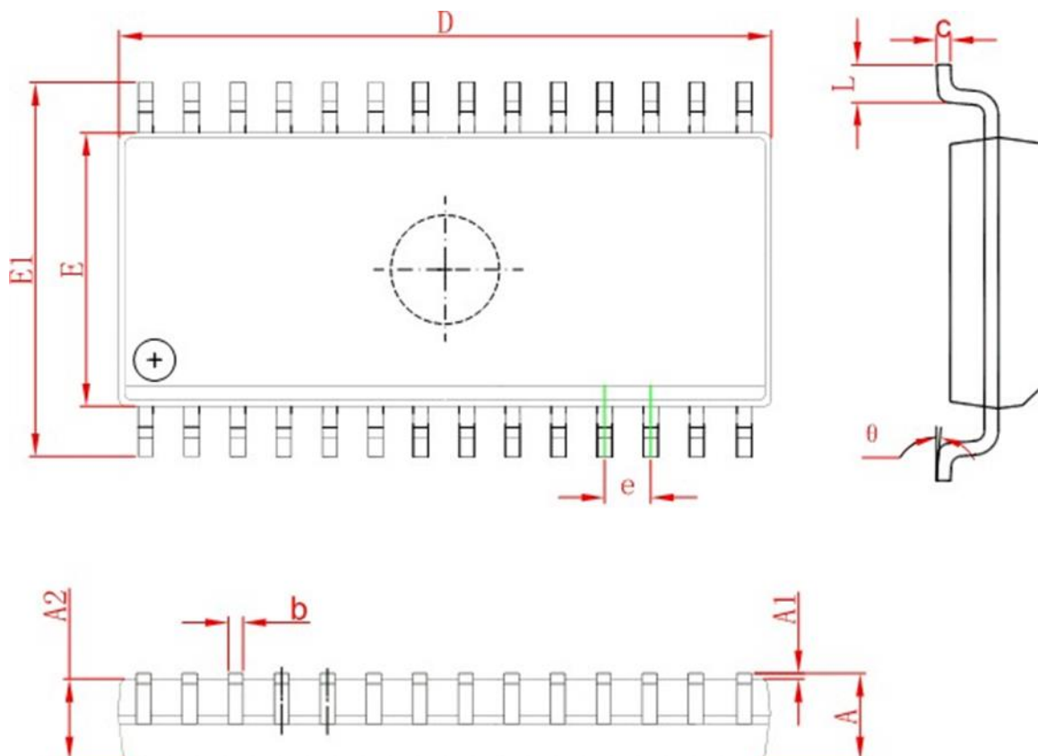
SOP-28(SOIC-28-300mil) 外形图与封装尺寸
