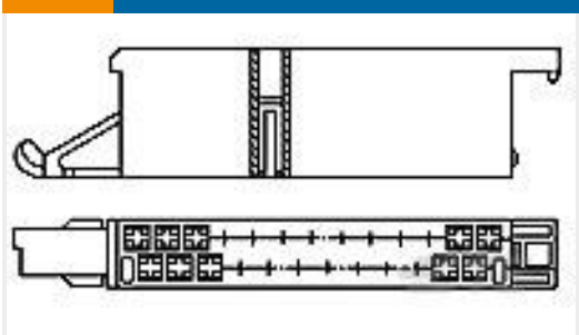
TE Part #925471-1 25P MINI TIMER HSG
