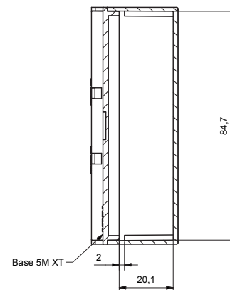
A-A (1:1)
