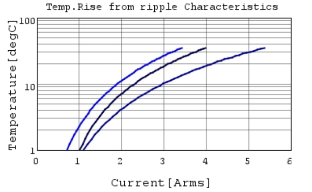
GCJ32DL8EL225KA07 Temp.rise — 100kHz
