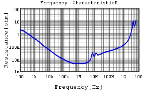
GCJ32DL8EL225KA07 R DCOV, 25degC
