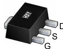
SOT-89 (SC-62)
