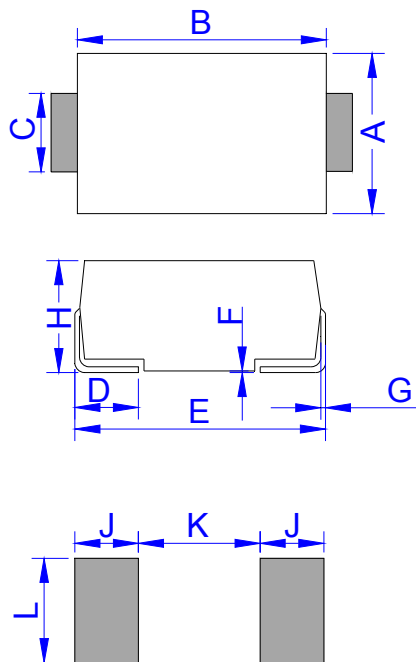
DO-214AB (SMC)
