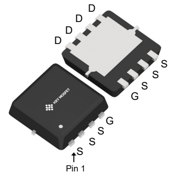
DFN3X3-8L (Power-33-8)
