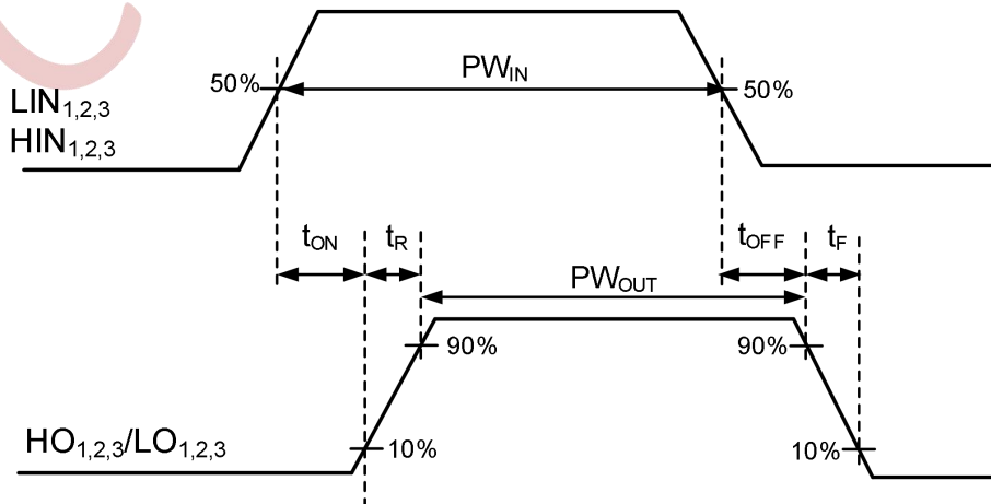
图 9-2 传输延时波形定义
