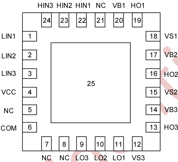
图 7-1 G2061Q QFN24 顶视图
