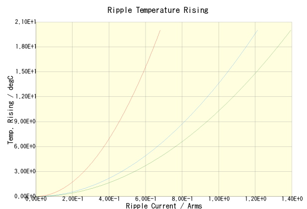
C0603X5R0J105M030BC(100kHz) C0603X5R0J105M030BC(500kHz) C0603X5R0J105M030BC(1MHz)
