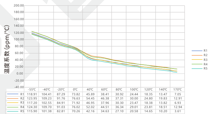
PEWM 系列 5930 规格 0.5mΩ 温度系数实测数据表
