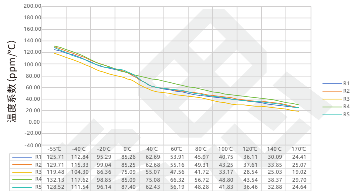
PEWM 系列 5930 规格 0.2mΩ 温度系数实测数据表
