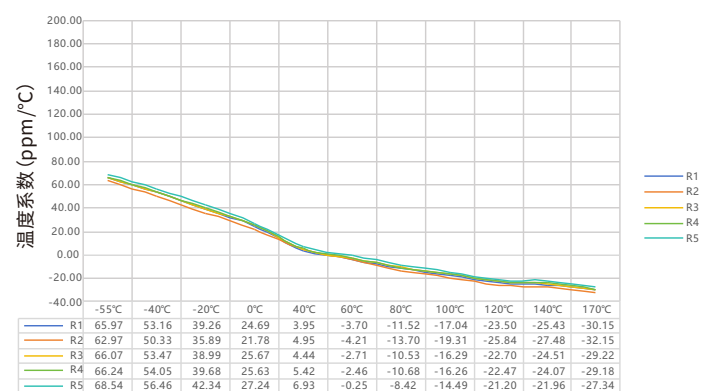
PEWM 系列 5930 规格 1.0mΩ 温度系数实测数据表
