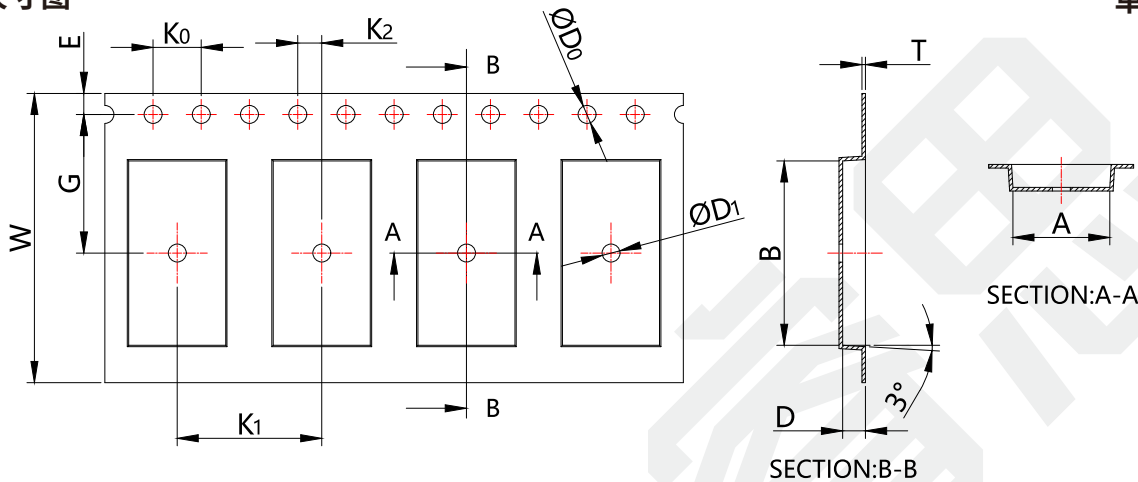
卷编带尺寸图
