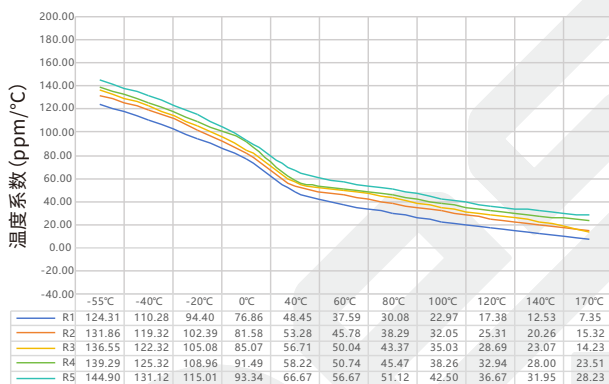
PEWM 系列 5930 规格 0.3mΩ 温度系数实测数据表
