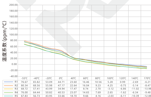
PEWM 系列 5930 规格 0.8mΩ 温度系数实测数据表
