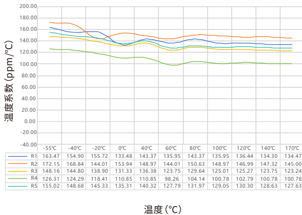
PEWM 系列 5930 规格 0.1mΩ 温度系数实测数据表
