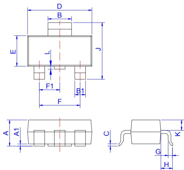
SOT-223-2L
