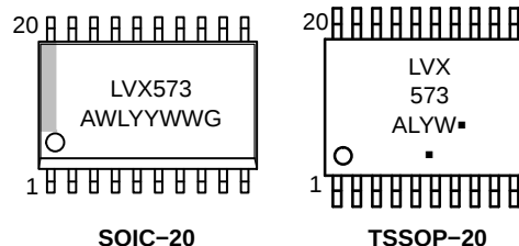
SOIC-20
