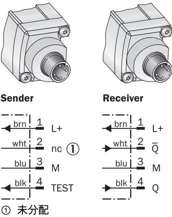
连接类型和连接图
