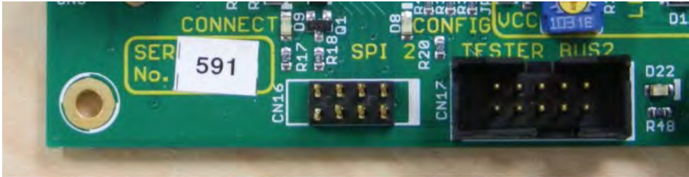
Fig 44. SPI 2 (Bus1 MCU) connector
