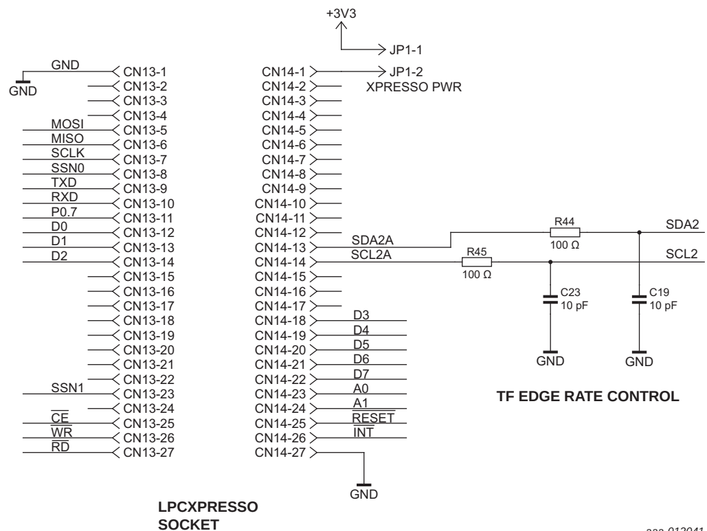
Fig 28. Bus2 master (LPC Xpresso)
