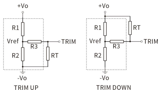
Trim 的使用电路(虚线框为产品内部)
