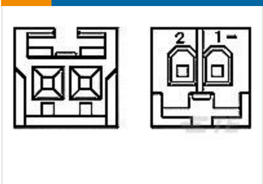
TE Part #172486-2 2P REC HSG CRIMP EI SER
