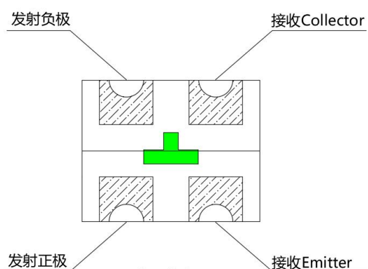
极性 Polarity
