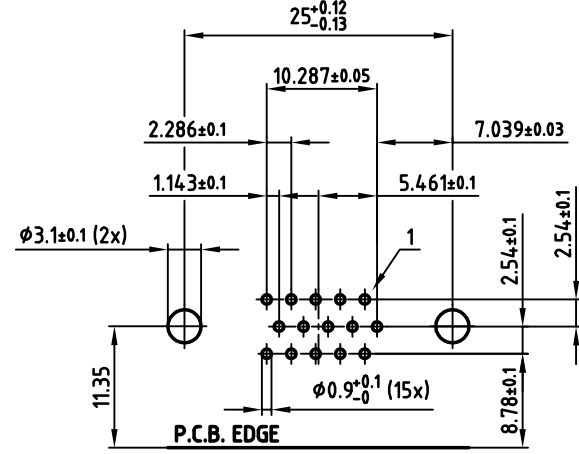
P.C.B. TOP SIDE
