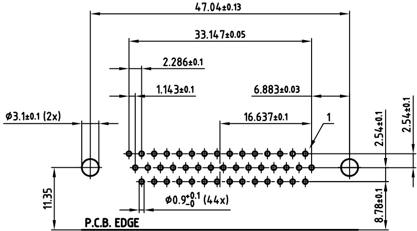
P.C.B. TOP SIDE
