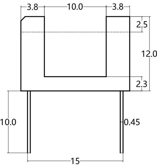
正面图
