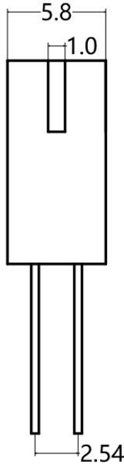
侧面图
