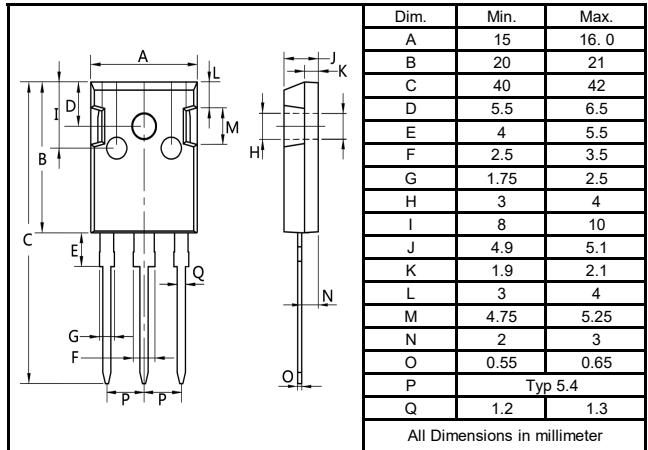
T0-247
