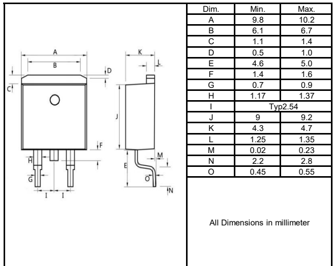
T0-263C
