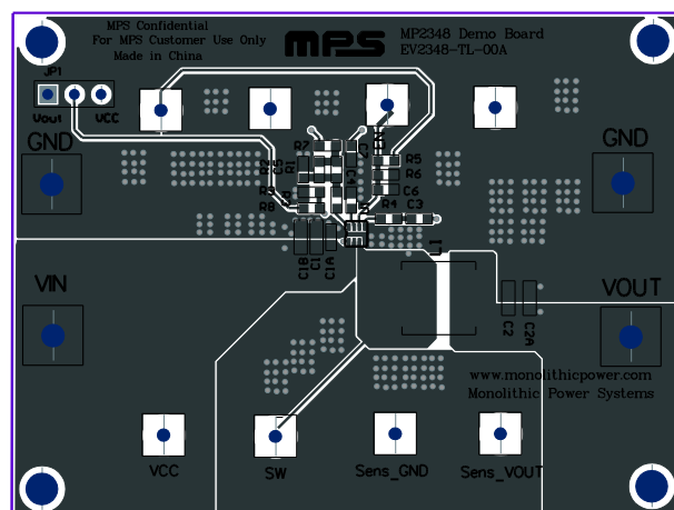
Top Layer
