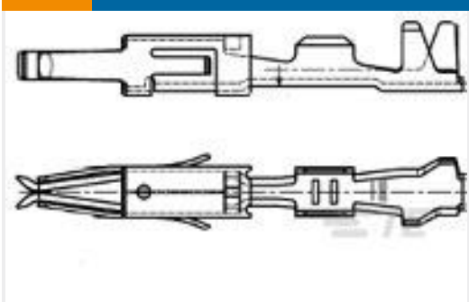
TE Part #962876-5 MT2 REC 1.6 Contact SWS Au
