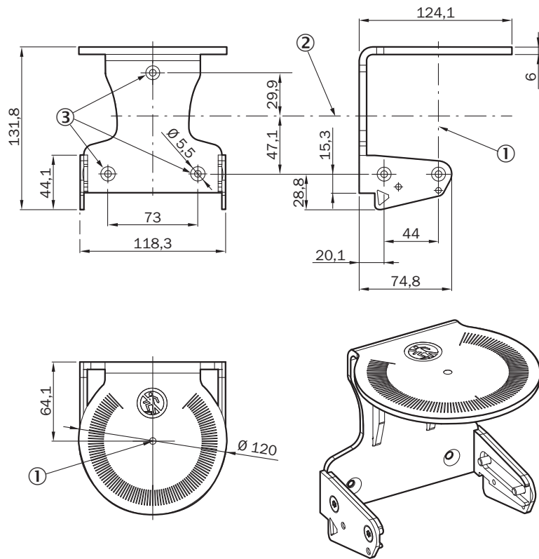
尺寸图 (尺寸单位: mm)
