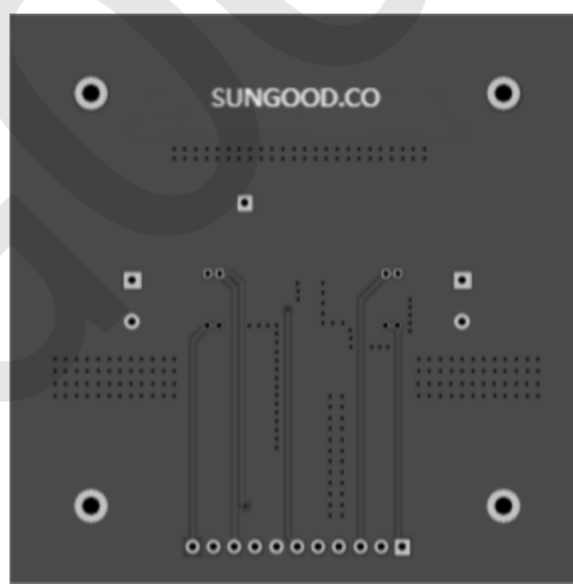
Bottom Layer
