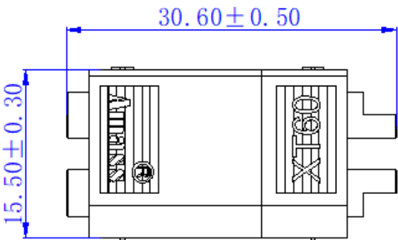
互配尺寸
