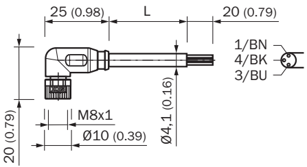
尺寸图 (尺寸单位: mm)
