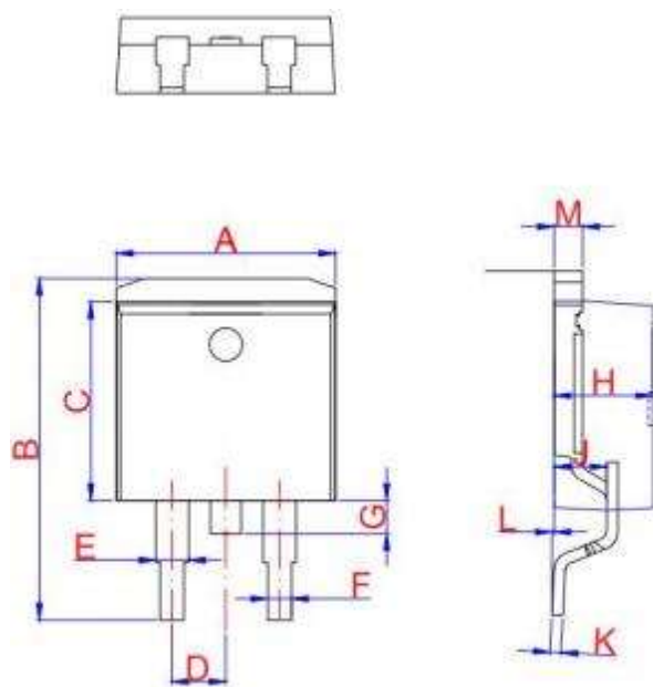
TO-263
