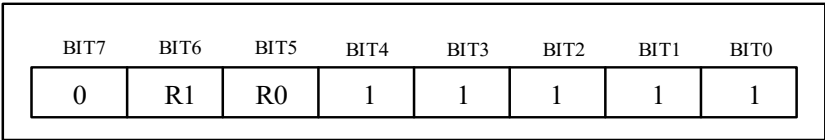
图 2-6 配置寄存器
