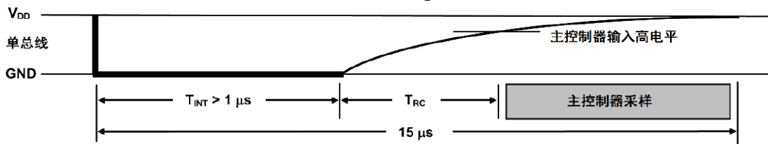
图 2-13 主控制器读取 1 时序
