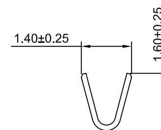
SEC:A-A
