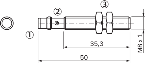
尺寸图 (尺寸单位: mm)
