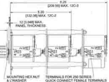
TYPES 12C-2, 12C-3
