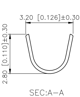
SEC:A-A
