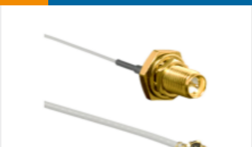
TE Part #CSI-RGFI-100-UFFR RP-SMA to U.FL/MHF1 100mm 1.13 OD
