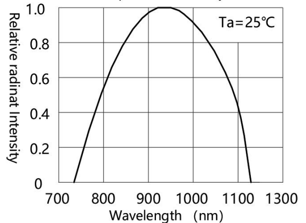
感应波长曲线图 Spectral Sensitivity
