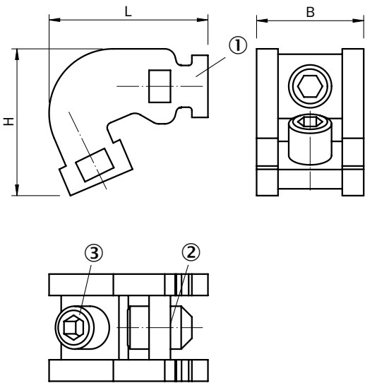
尺寸图 (尺寸单位: mm)
