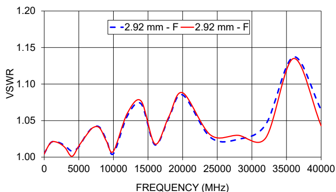
KFFL-KF50+ VSWR
