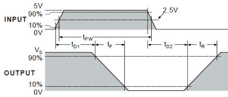
图 9-1 输入输出(A 通道反相)波形图
