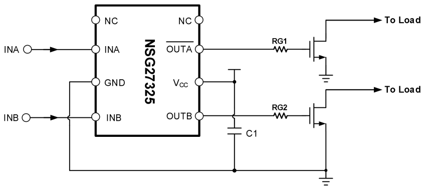
图 10-2 NSG27325 反相典型应用电路图
