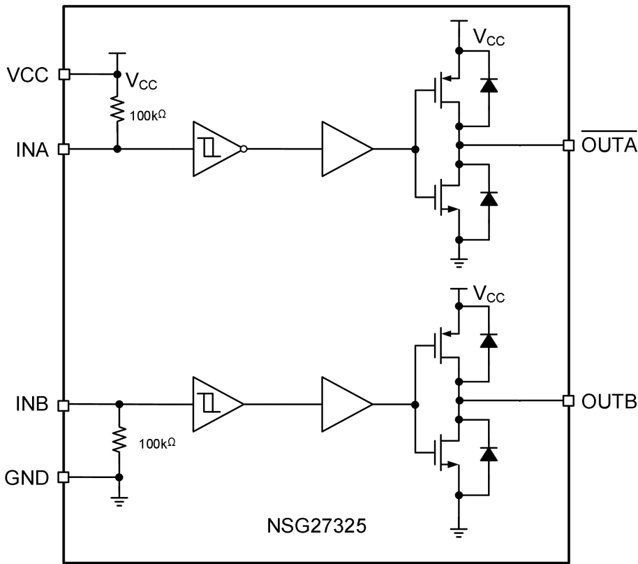
图 10-1 NSG27325 功能框图
