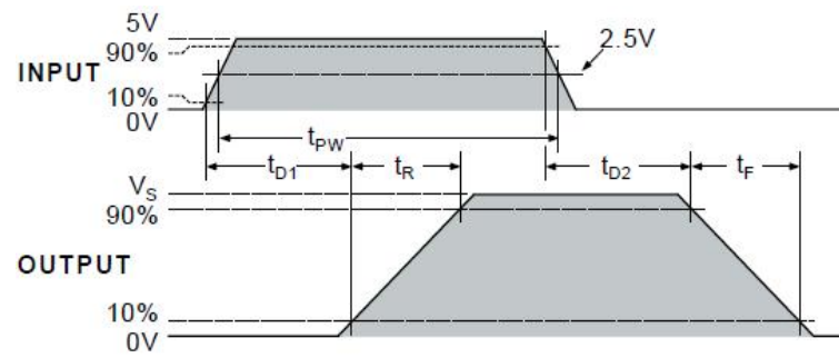
图 9-2 输入输出(B 通道同相) 波形图
