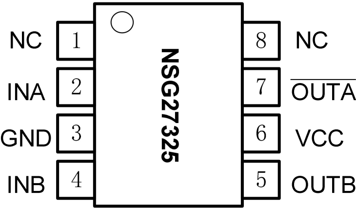
图 7-1 8-脚 SOP8 顶视图
