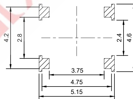
PCB. 焊接图
