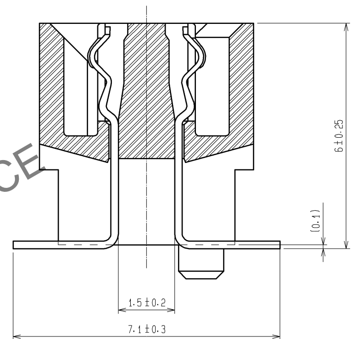
A-A (10:1)
