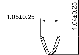
SEC:B-B
