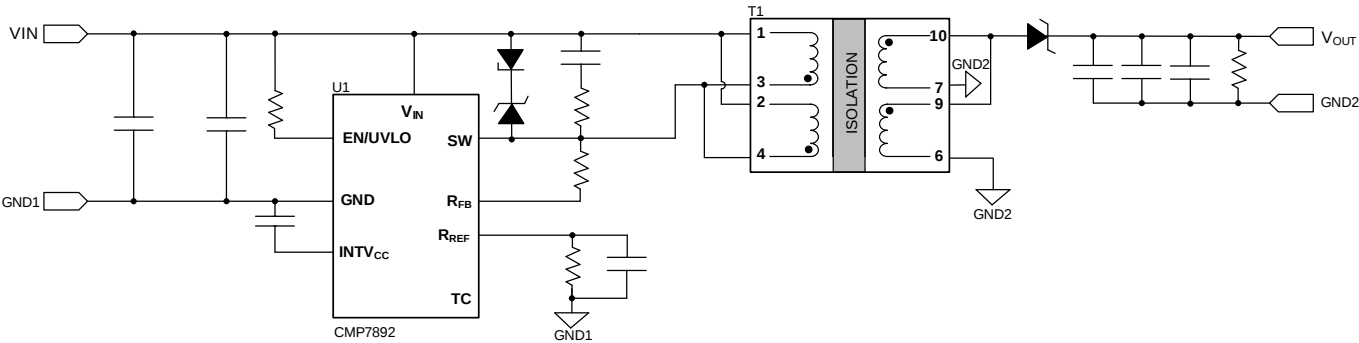
图1. CMP7892 单路输出
