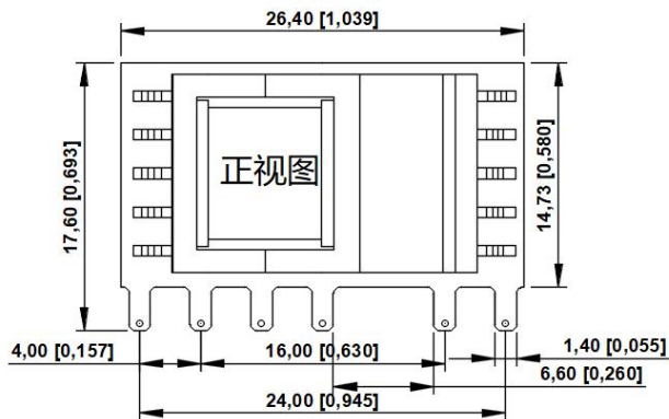
外观尺寸图
