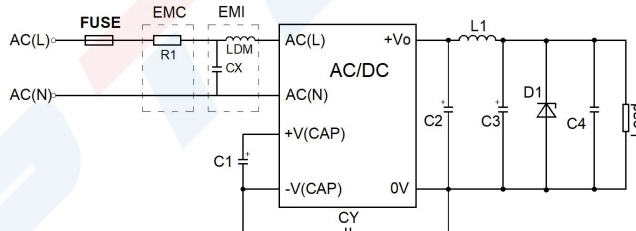
推荐电路 4
