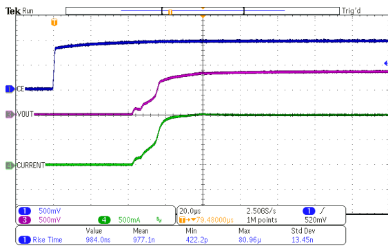
SUL6001D8-18
