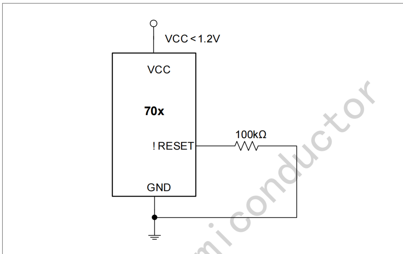
图 7 确保!RESET 正常工作电路
