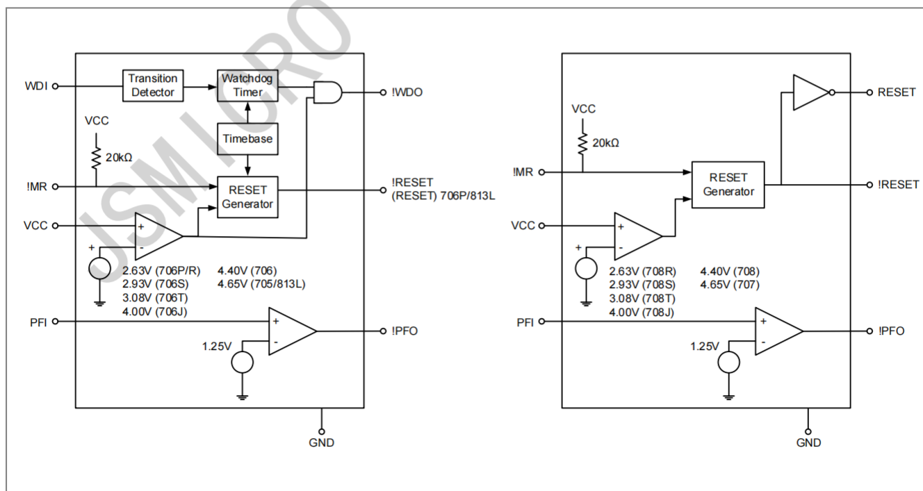
图 1 706P/R/S/T/J, 708R/S/T/J, 705/6/7/8, 813L 的结构示意图
