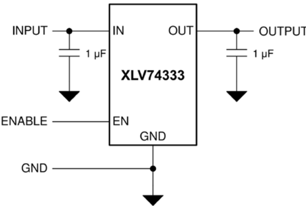
电路连接图
