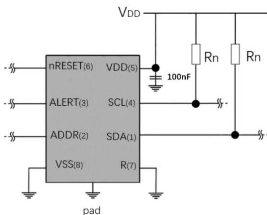
图 5 典型应用图
