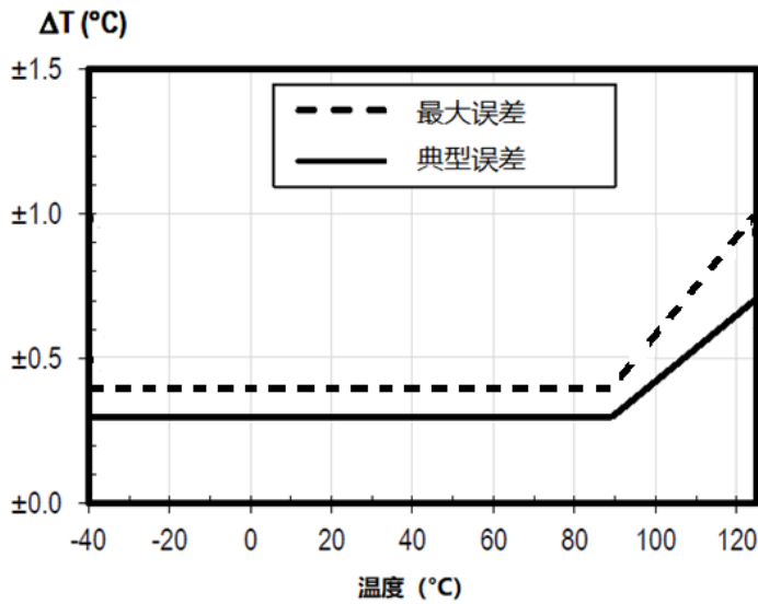
图 4 GXHT30 温度误差图
