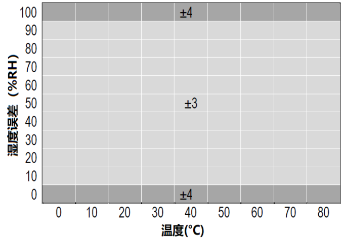
图 3.1 不同温度条件下 GXHT30 的误差
