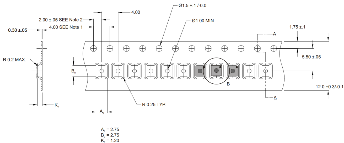
图 9 芯片运输用编带尺寸说明
