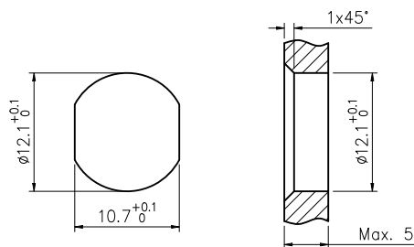
面板开孔尺寸
