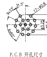
P.C.B 开孔尺寸
